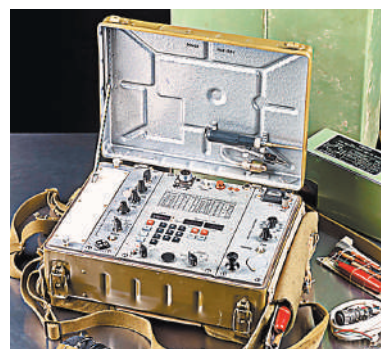
Сообщения с радиостанции «Стриж» отправлялись в кодированном виде группами по 5 цифр. Фото Jürgen Vogel/LVR-LandesMuseum Bonn
